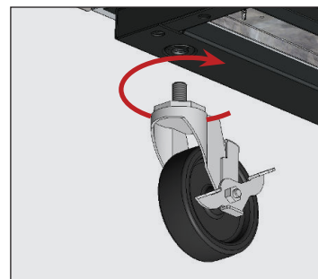
Fig. 8. Atornille las ruedecillas en los orificios roscados.
