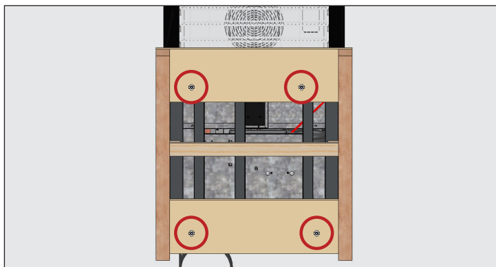
Fig. 2. Ejemplo de ubicaciones de los pernos de transporte.
