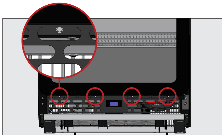
Fig. 3. Retire los pernos de la rejilla delantera para acceder a los pernos de transporte.
