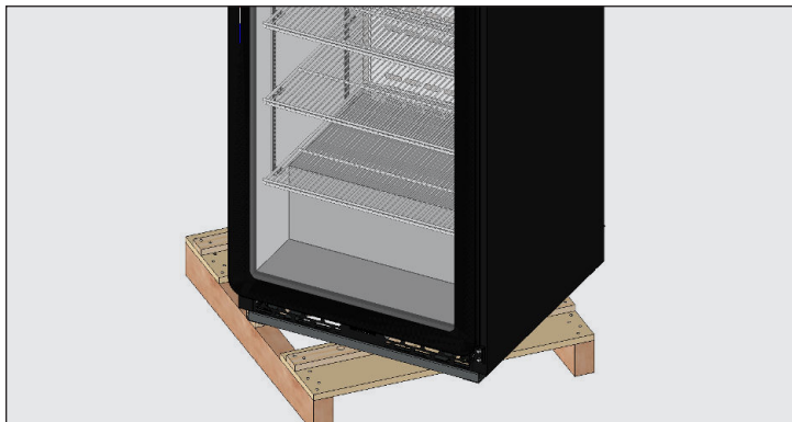
Fig. 4. Ruotare l'elettrodomestico sul pattino. Quando si solleva l'unità, non utilizzare banconi di lavoro, sportelli/cassetti o griglie come punti di sollevamento.
