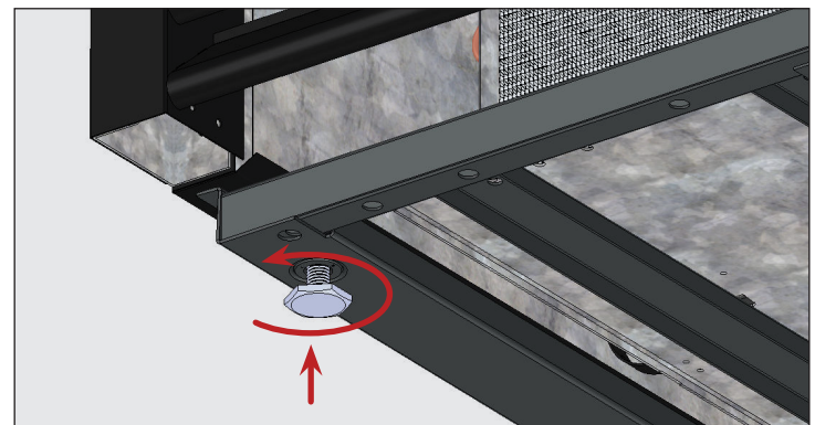
Fig. 3 Girare le viti di livellamento in senso antiorario per sollevare l'elettrodomestico.
