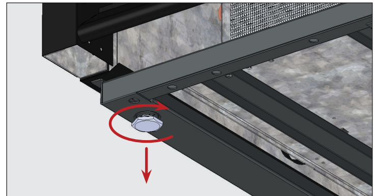
Fig. 2 Girare le viti di livellamento in senso orario per abbassare l'elettrodomestico.
